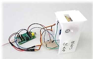
「単三電池仕分け機」 福井県立高志中学校 1年 藤本 理史
